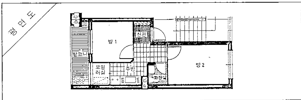
임대아파트 평면도
